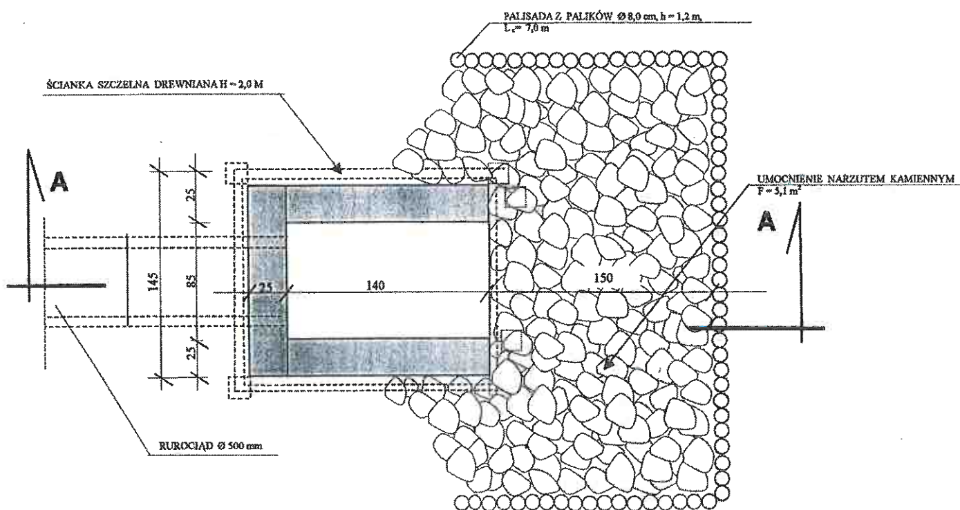
WYLOT KANAŁU DESZCZOWEGO – PRZEKRÓJ PODŁUŻNY 1 : 25
