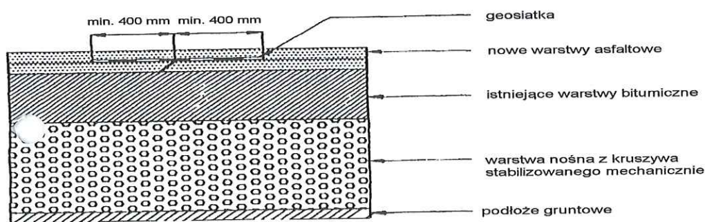
Rys. 4. Wzmocnienie nawierzchni asfaltowej w strefie zmiany konstrukcji nawierzchni
