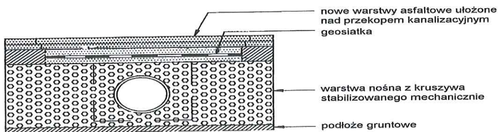
Rys. 2. Wzmocnienie nawierzchni asfaltowej w strefie zmiany nośności podłoża gruntowego
