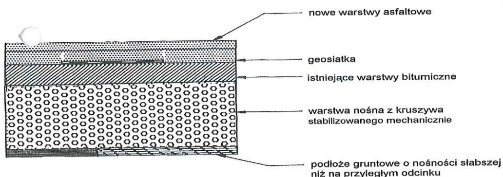
Rys. 3. Wzmocnienie nawierzchni asfaltowej w strefie spiny roboczej
